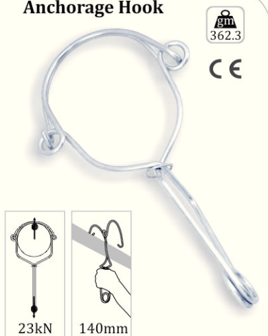
Ref. PN 141 Anchorage Hook
